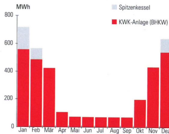
Effizienzbeispiel Kraft-Wärme-Kopplung
